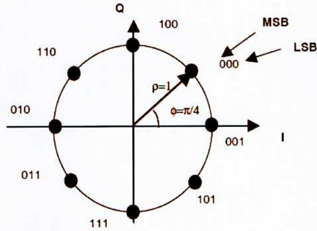
图 10 8PSK 星座图
