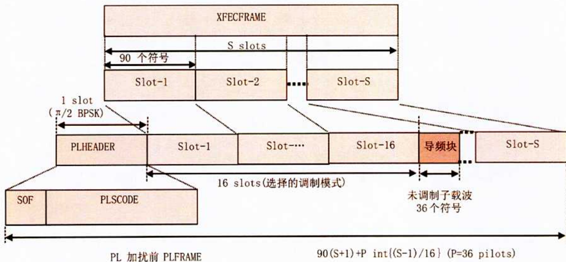
图 13 PLFRAME 格式
