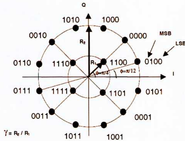
图 11 16APSK 星座图
