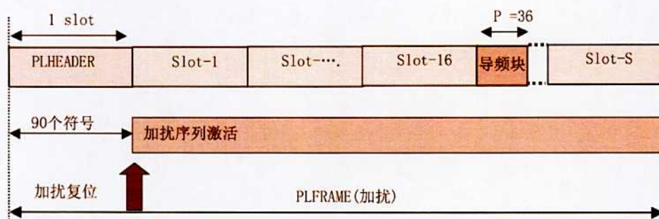
图 15 PL 加扰
