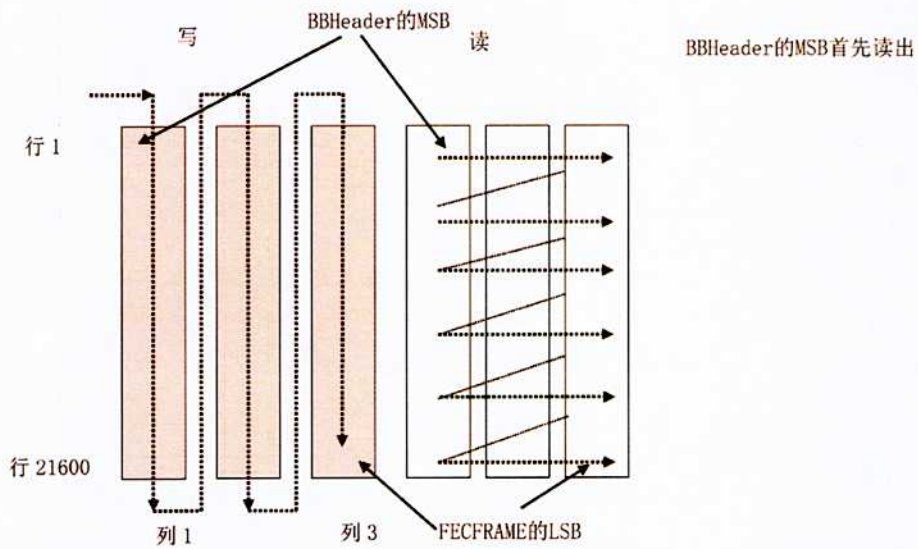
图 7 8PSK 和标准长度 FECFRAME 的比特交织方案（除 3/5 码率外的所有码率）
