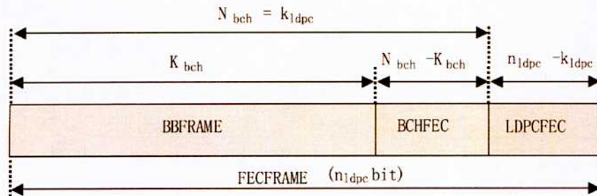
图 6 比特交织前的数据格式
