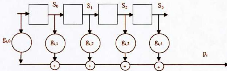
图 C.2 卷积码编码框图
