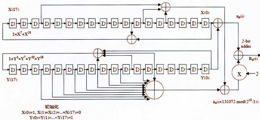
图 16 n=0 时 PL 扰码生成器的配置框图
