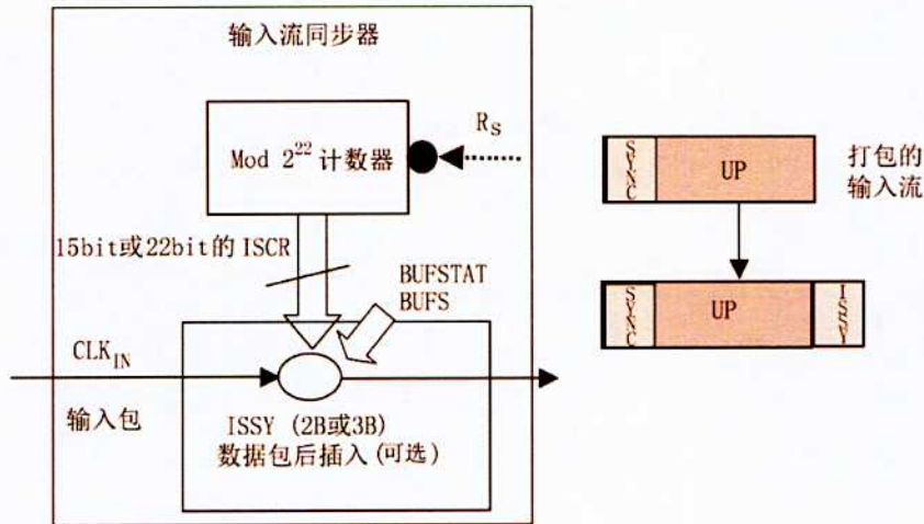
图 A. 2 输入流同步器模块框图
