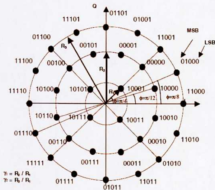
图 12 32APSK 星座图
