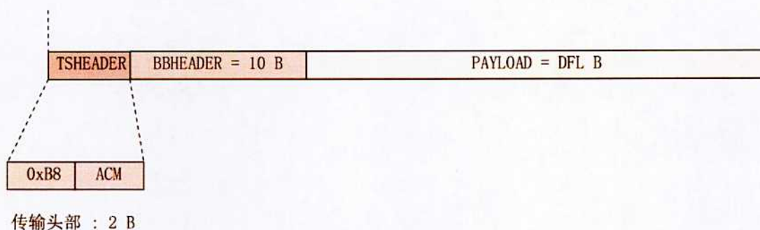
图 B.2 模式适配输入接口的模式适配格式
