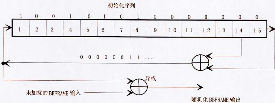
图 5 PRBS 实现框图
