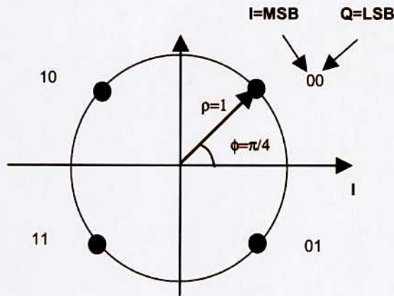
图 9 QPSK 星座图
