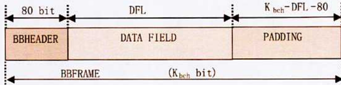
图 4 流适配器输出端 BBFRAME 格式
