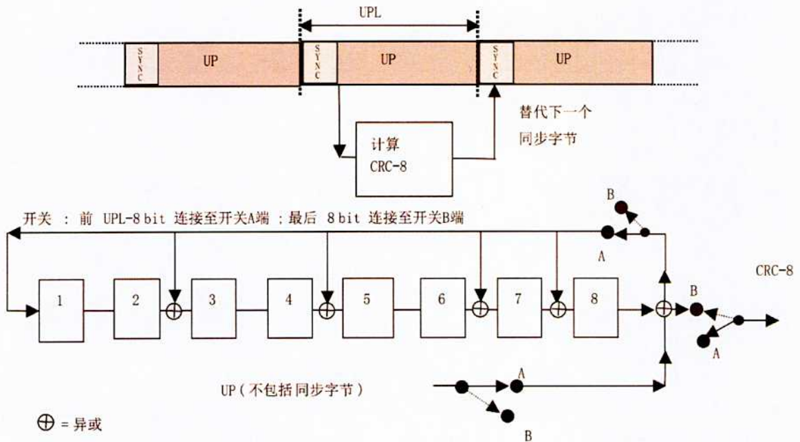
图 2 CRC-8 实现框图
