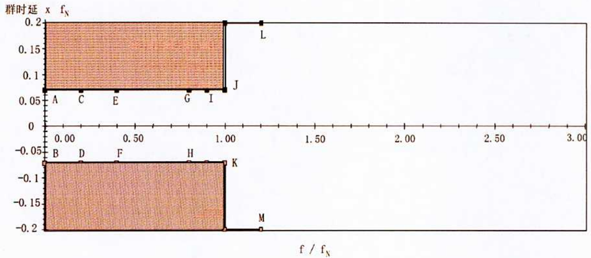
图 F.2 调制器滤波器群时延模板
