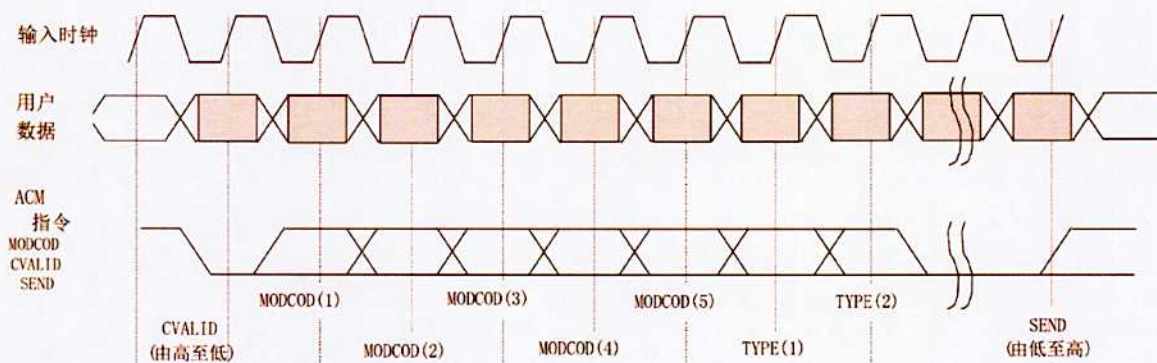
图A.1 ACM指令示例（串行格式）
