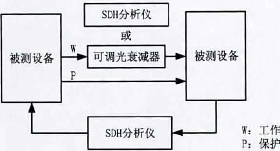
图9 保护倒换测量框图
