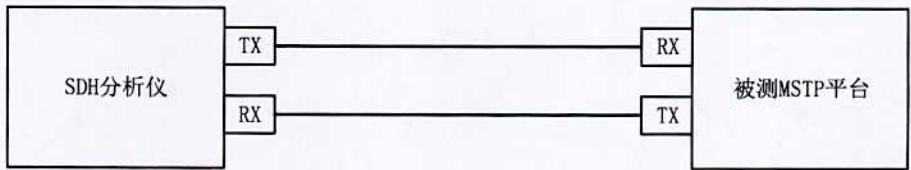
图6 输入口允许频偏测量框图
