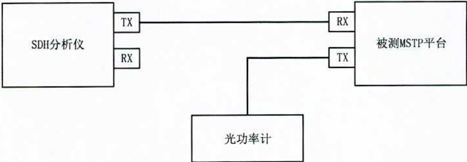
图2 平均发送光功率测量框图
