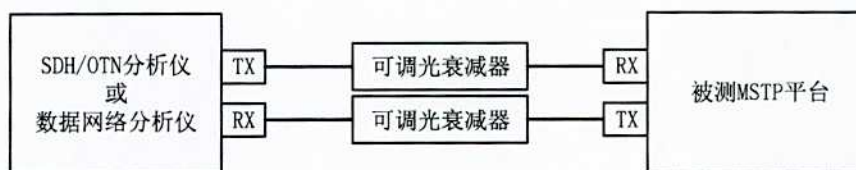
图8 误码/丢包性能测量框图
