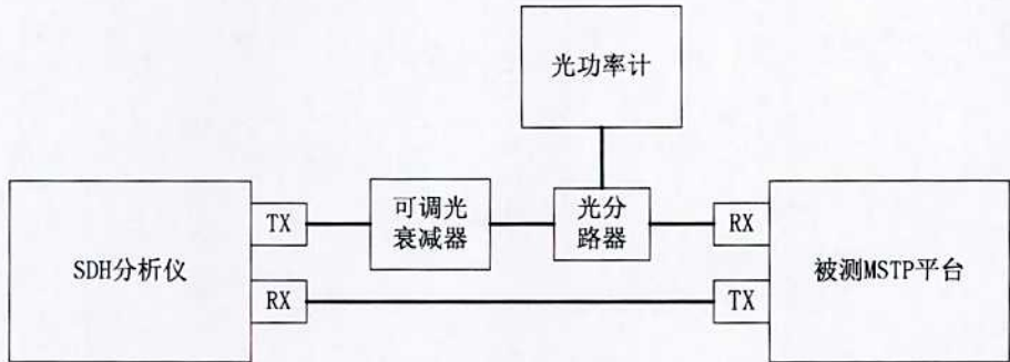
图5 接收机灵敏度测量框图
