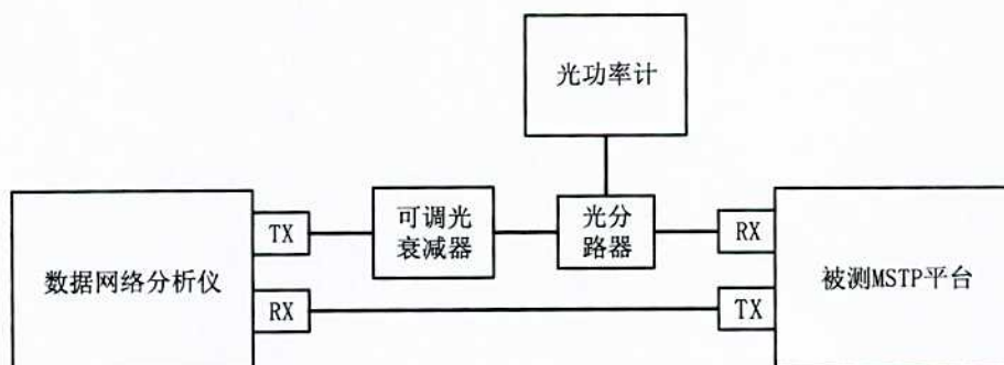
图13 接收机灵敏度测量框图
