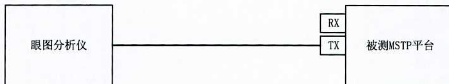
图11 消光比测量框图
