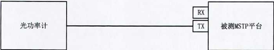
图10 平均发送光功率测量框图
