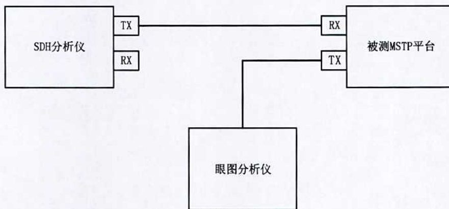
图3 发送信号波形、消光比测量框图
