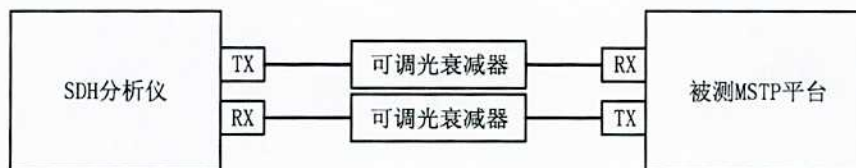
图7 输出抖动测量框图
