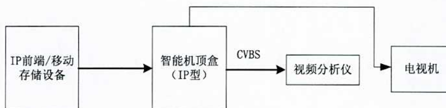
图4 复合视频输出测量框图
