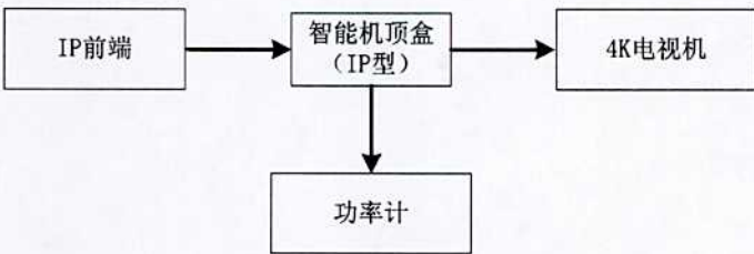
图 7 整机待机功率测量框图
