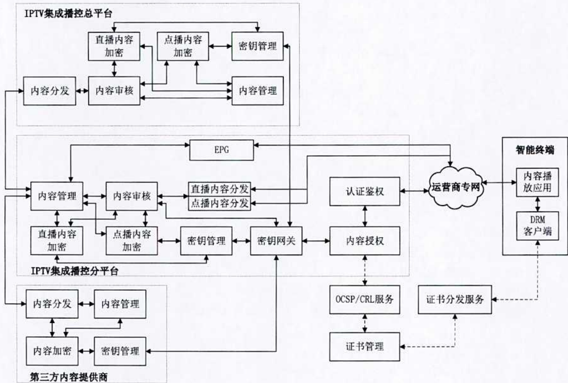
图1 IPTV DRM系统集成框架
