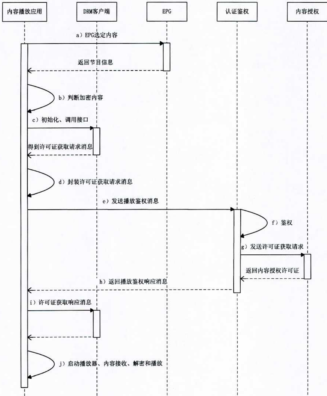
图2 IPTV 智能终端播放加密内容流程
