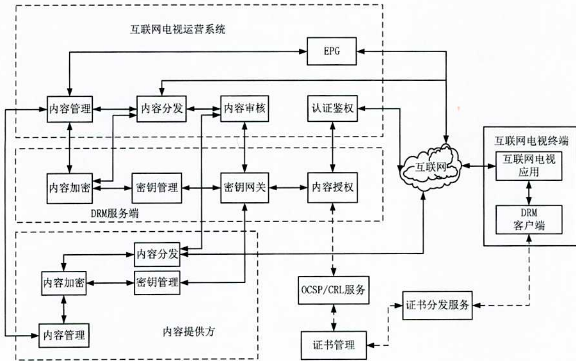
图1 互联网电视数字版权管理系统集成框架
