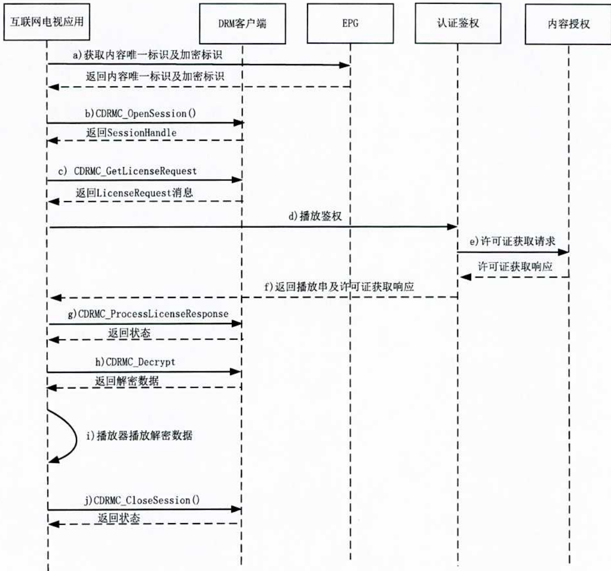
图2 互联网电视终端应用播放加密内容流程
