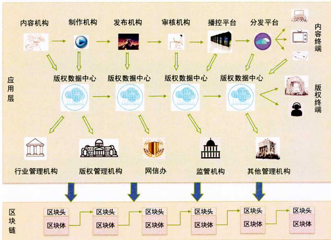
图 6-1 媒体内容全流程版权保护和安全共享架构
