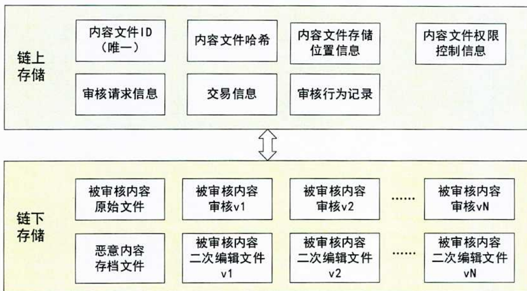
图 1 内容审核分布式存储架构
