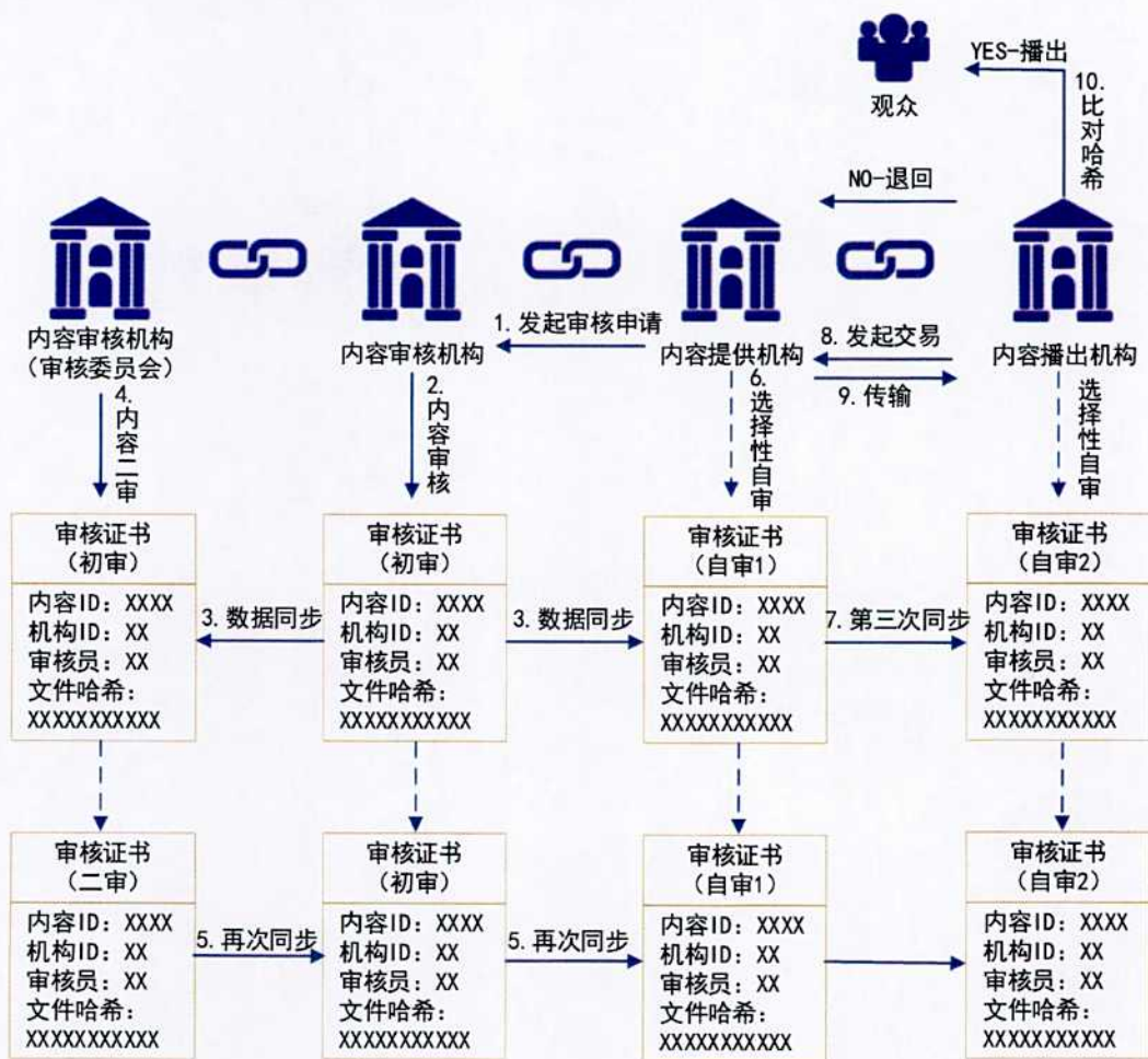
图 5-3 上级二审流程
