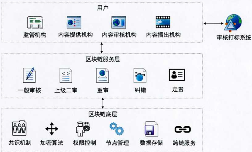
图 3-1 基于区块链的内容审核方案架构
