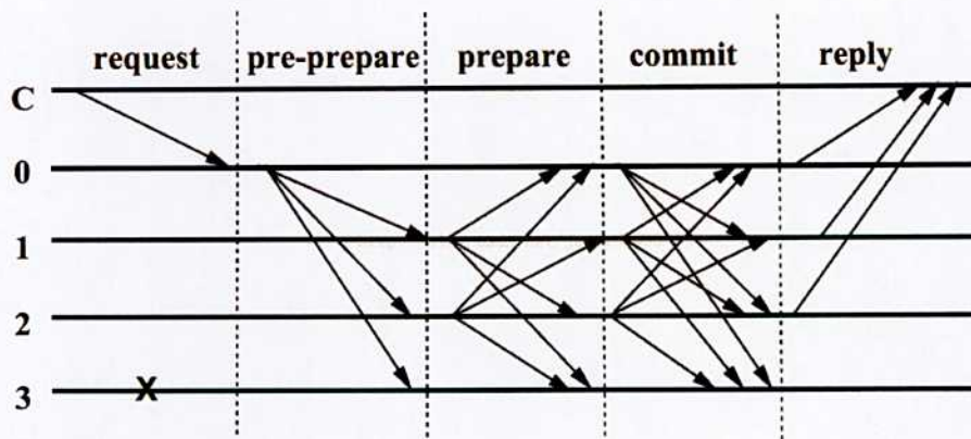
图 4-3PBFT 共识算法
